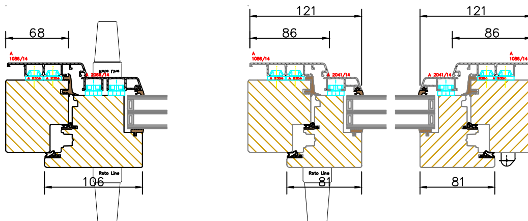
Cas d'une poignée traversante avec cylindre. 1 point de verouillage
