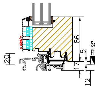
Cas d'un seuil encastré pour norme handicapée
